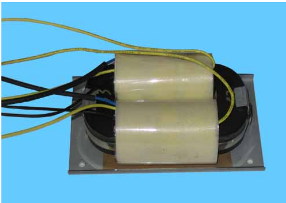
用于靜電音箱的 C 型音頻變壓器
