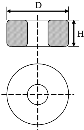
環型燈飾變壓器外形尺寸圖
