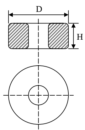
環型電源變壓器外形尺寸圖
