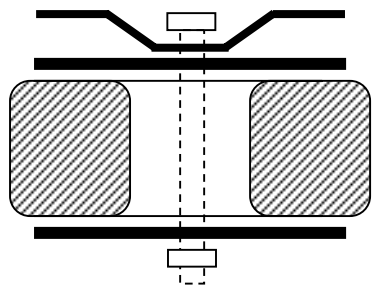
環型電源變壓器安裝示意圖
